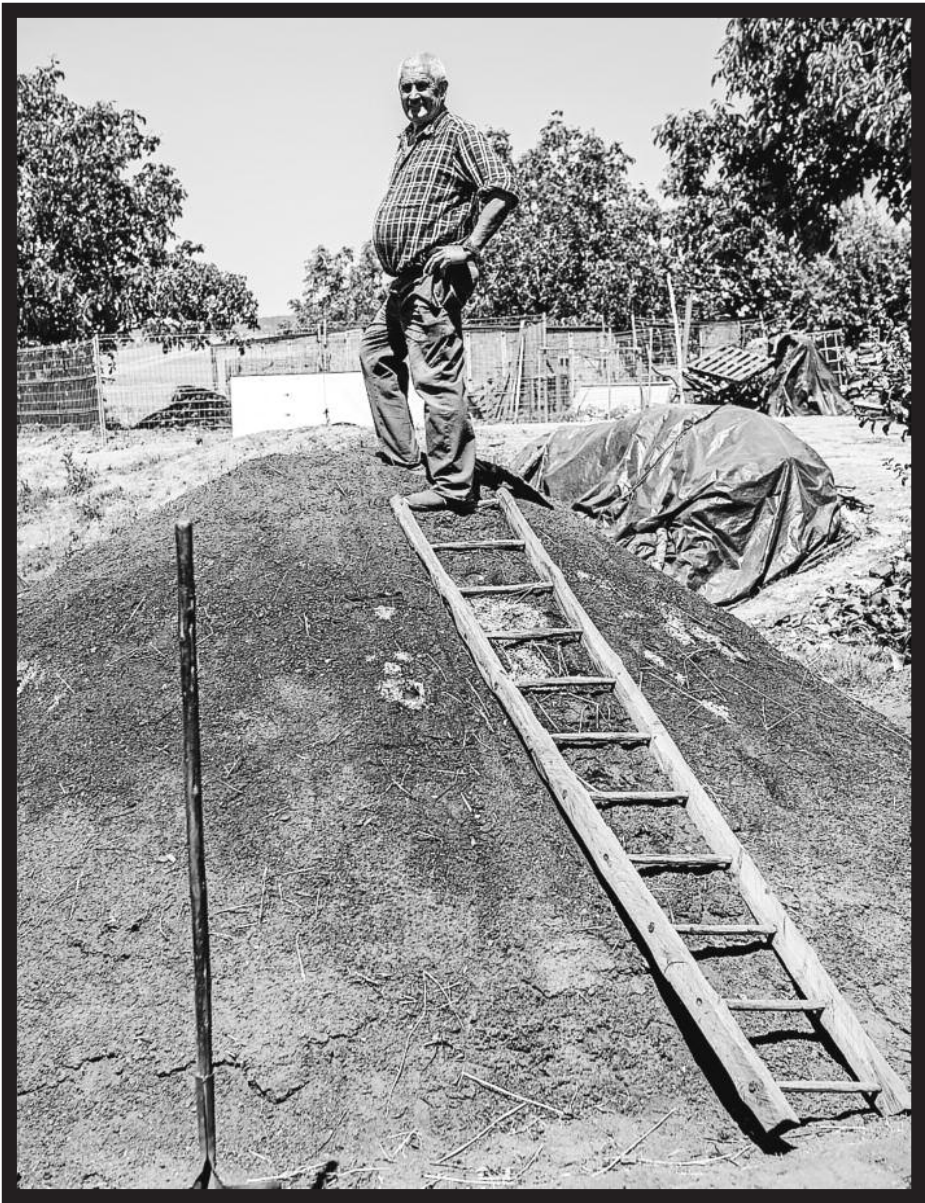
Egoste prozesua amaitutakoan, txondorra hustu egin behar da. Ikatza lortzea atsegina da, baina egitura desegitea lan gogorra dela dio Remirok. Juanan RUIZ | ARGAZKI PRESS
